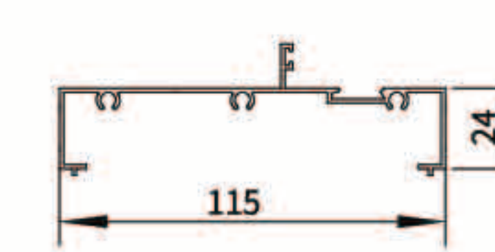
包边 TOP VENT
