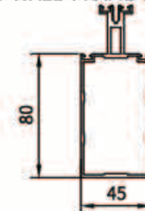
横梁 CURTAIN WALL FRAME-HORIZONTAL
