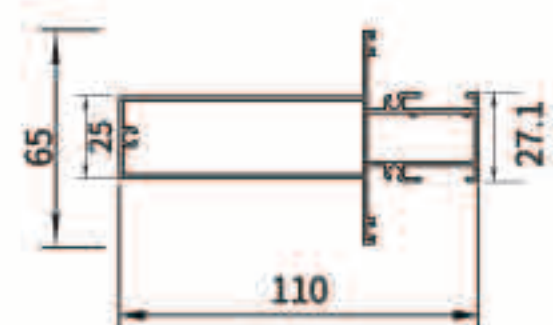
三轨边窗 VENT TRANSOME
