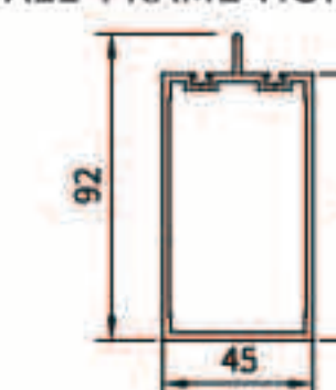
横梁 CURTAIN WALL FRAME-HORIZONTAL
