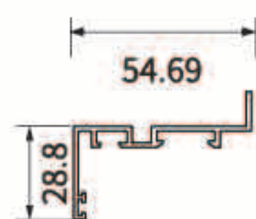
收口 ADAPTOR
