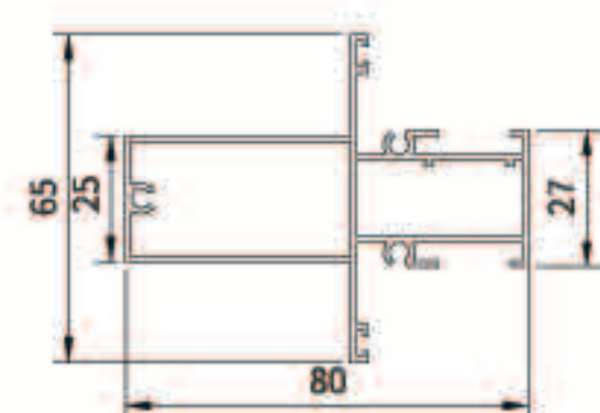
二轨中柱 TRANSOME
