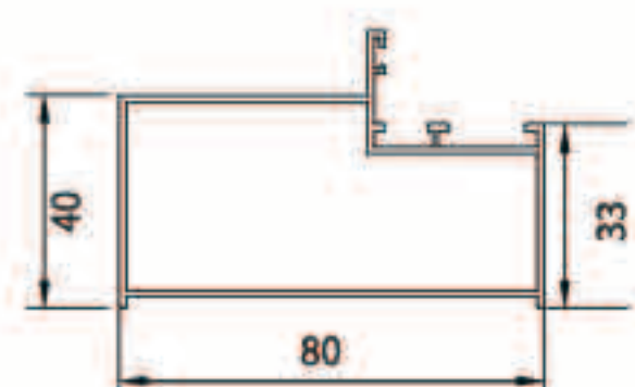
外边框 DOOR FRAME
