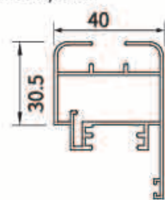
门扇料 DOOR SHUTTER/OUT
